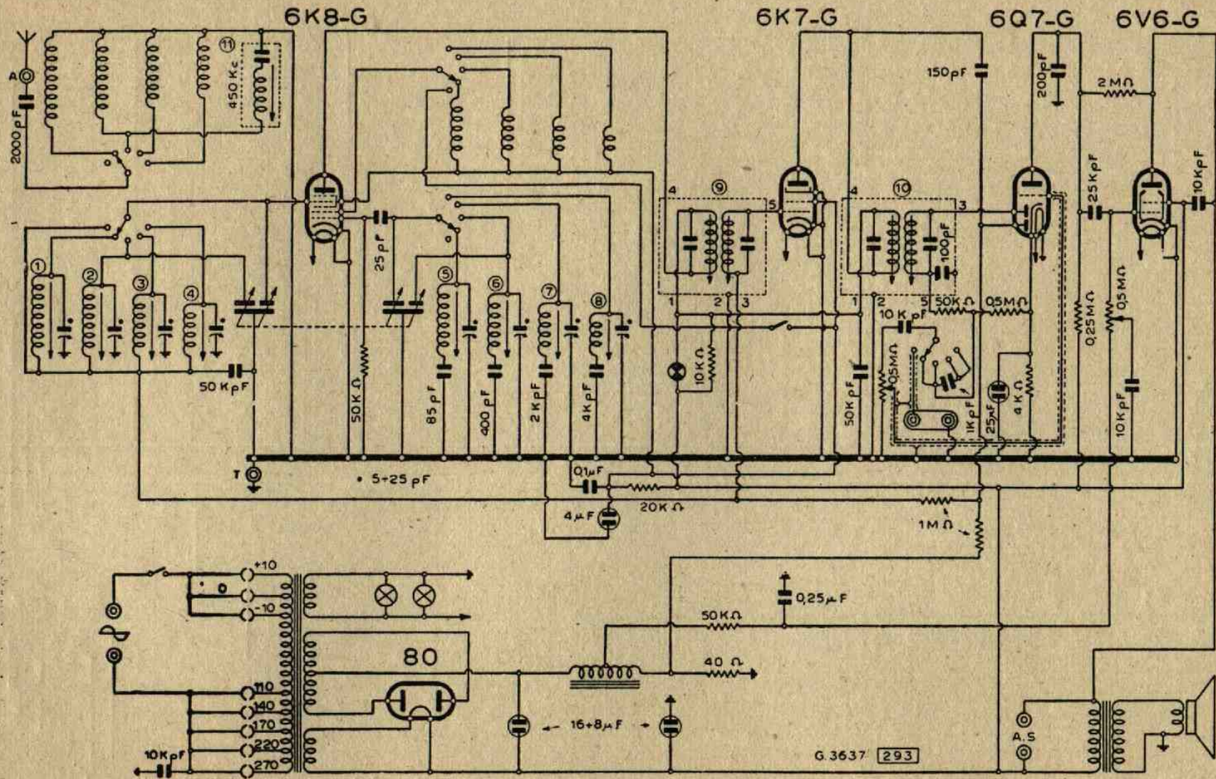
Lo schema elettrico del Quadri-Unda 541 con cui si realizza anche il radiofonografo Q. U. 543.
